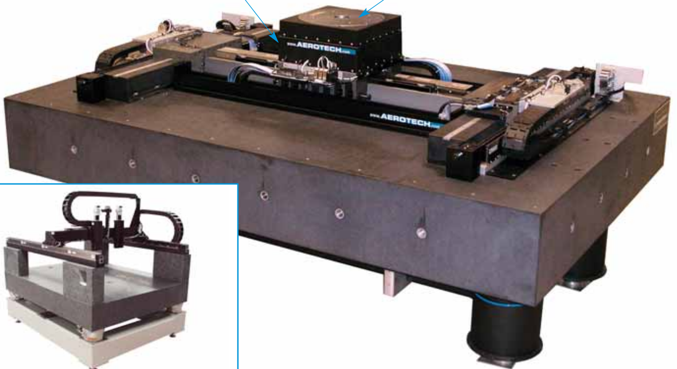
Flachbildschirm-Prüfstation in Portalbauweise mit einem Verfahrensweg von 1800 x 800 x 200 mm.
